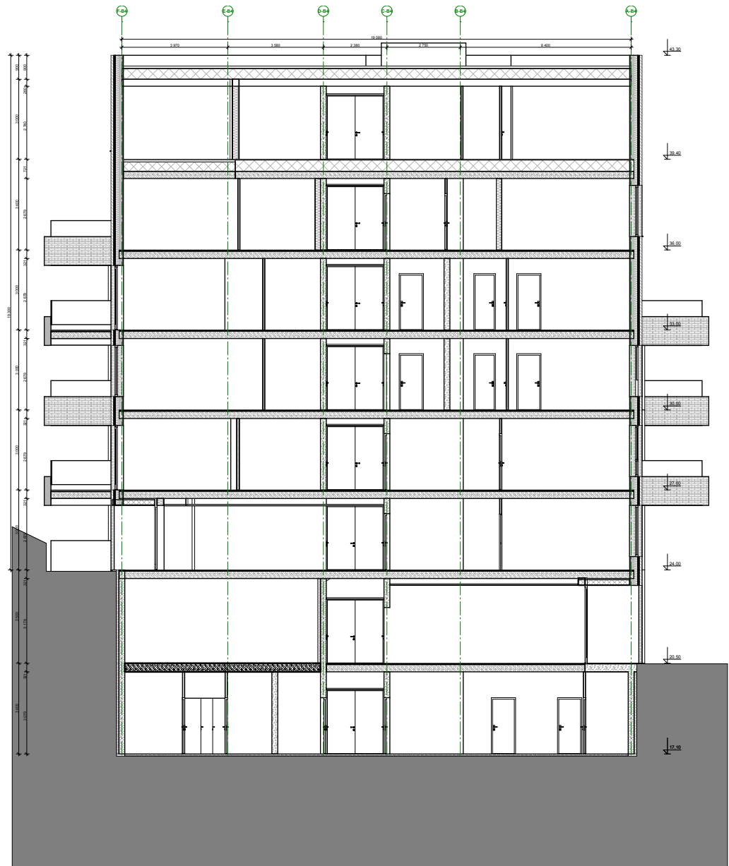
Snitt B-B
