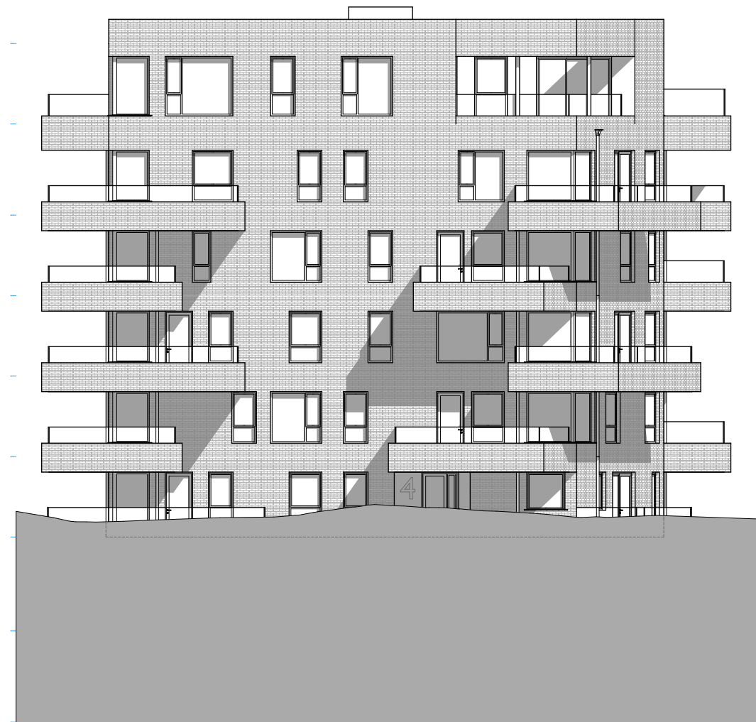
Sørvestre fasade
