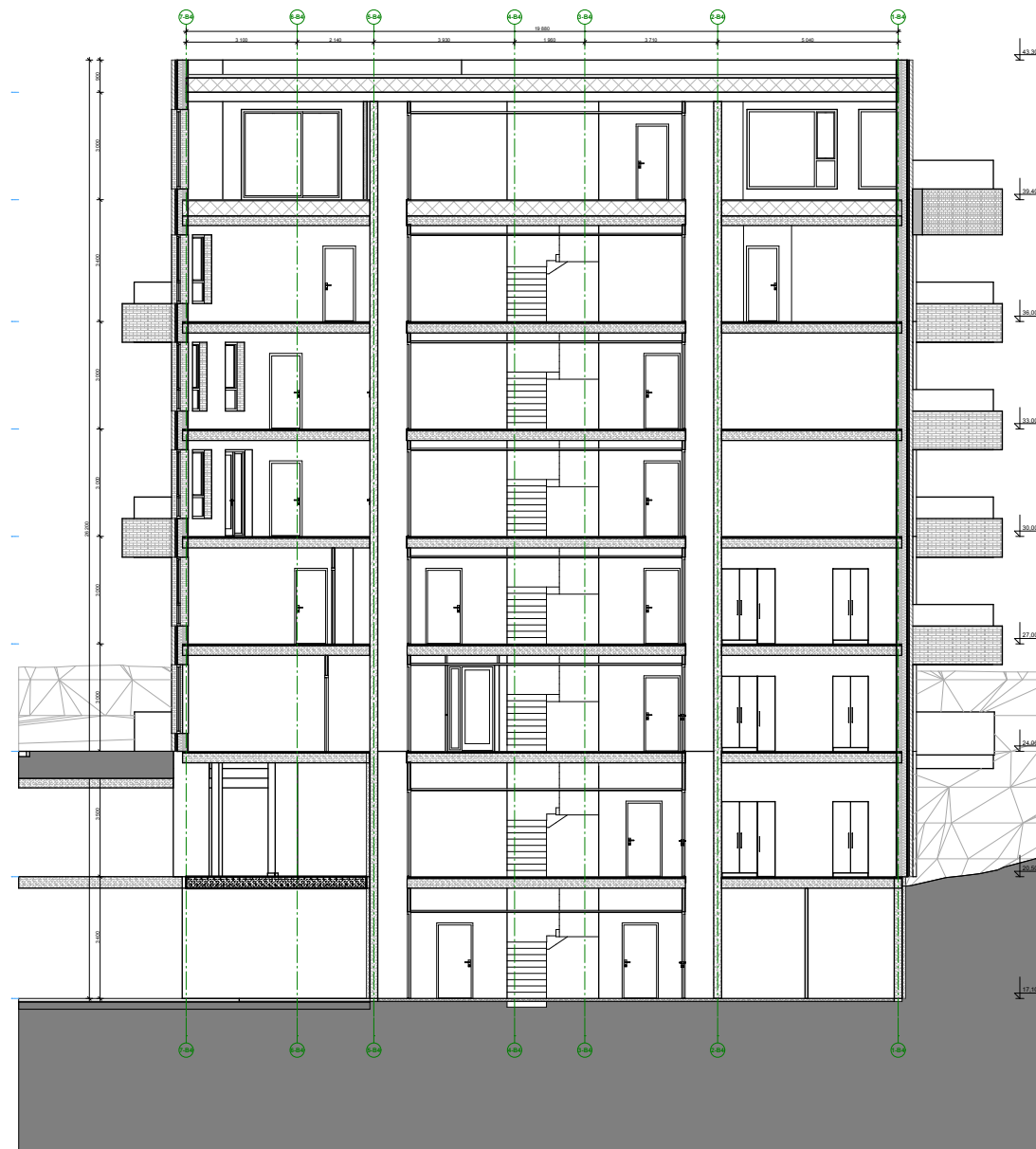
Snitt A-A
